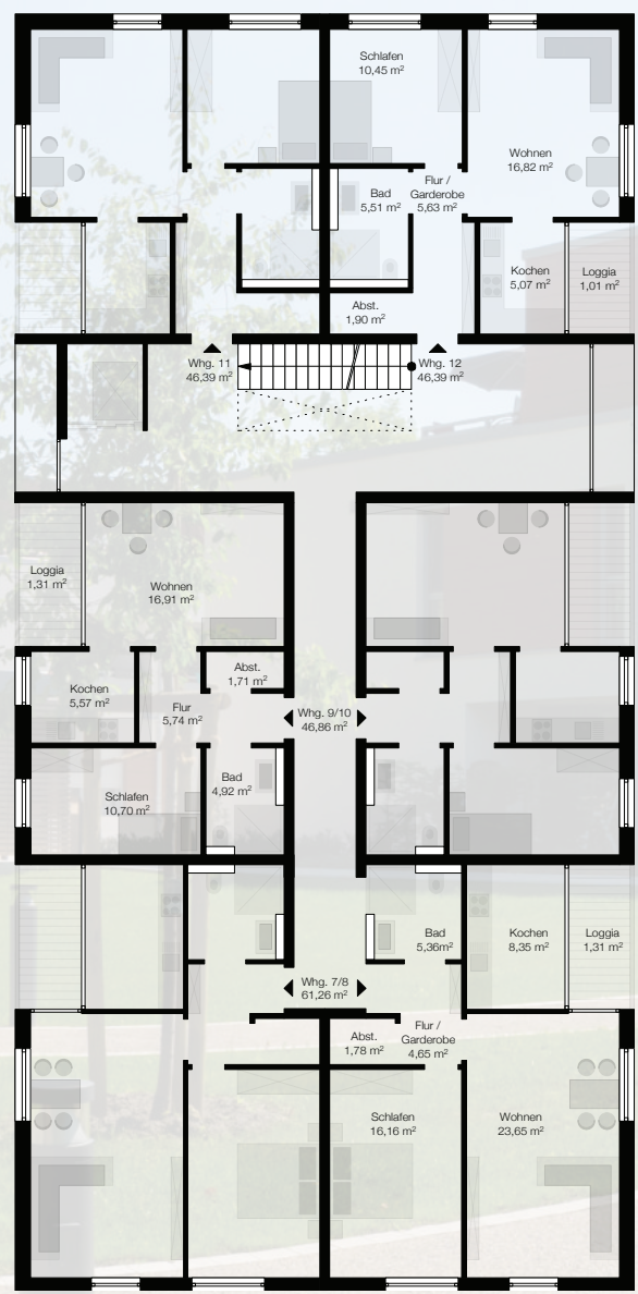
Obergeschoss Jägerallee M. 1:200
