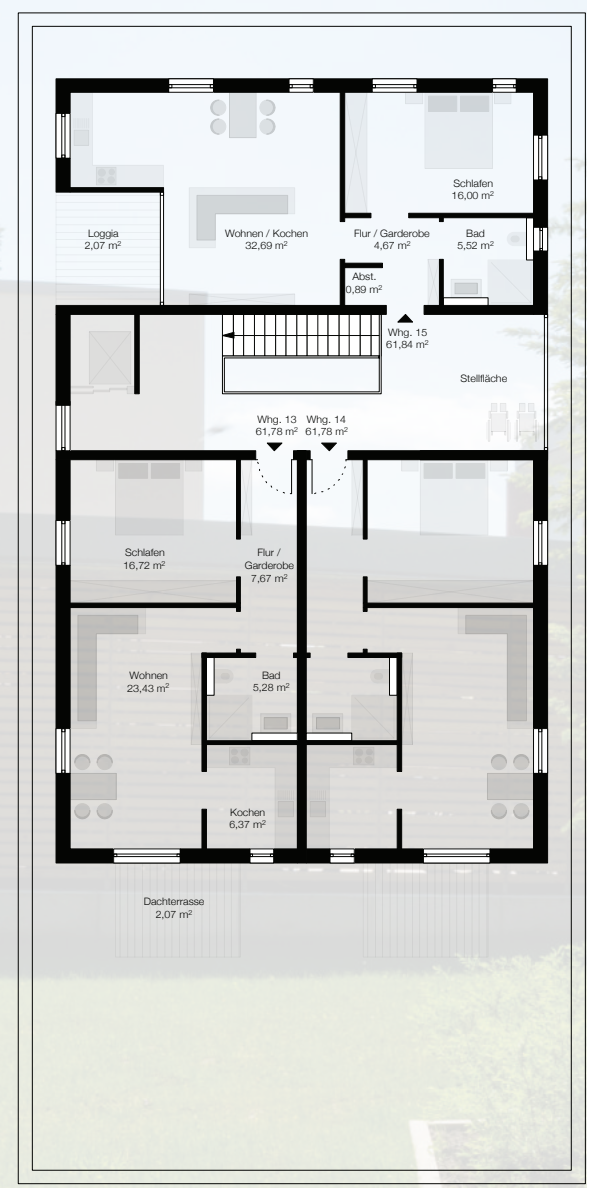
Staffelgeschoss Jägerallee M. 1:200
