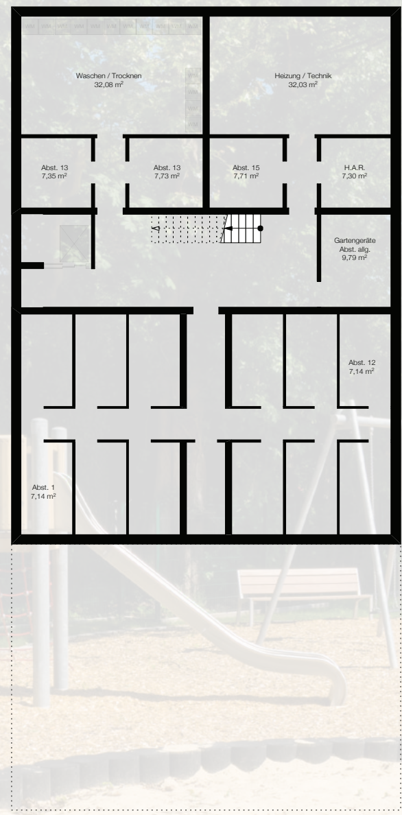
Untergeschoss M. 1:200
